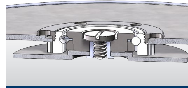
Roulement de masse oscillante standard en coupe Standard oscillating mass bearing in cross-section
