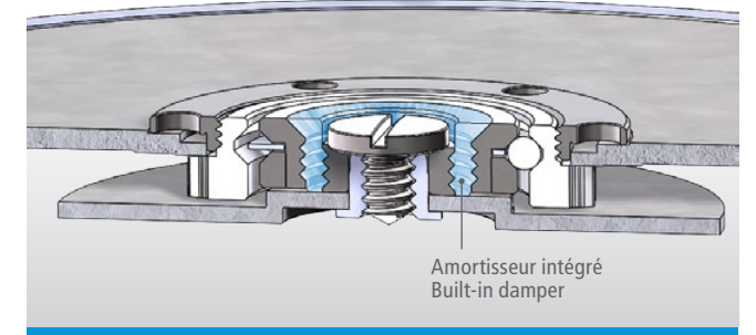
Roulement ActiVib en coupe ActiVib bearing in cross-section
